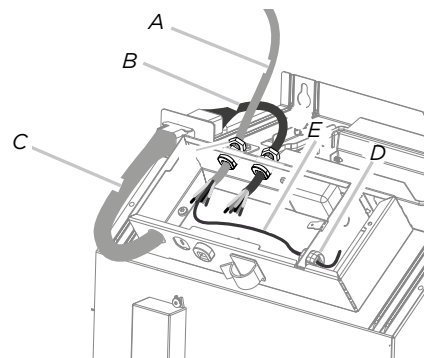
A. Conduit de câblage du ventilateur en ligne (non inclus) B. Connecteur 9 fils C. Insert de capot D. Range Hood strain relief E. Vis décharge de traction
