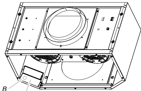
A. Boîtier de raccordement électrique B. Opércule arrachable
