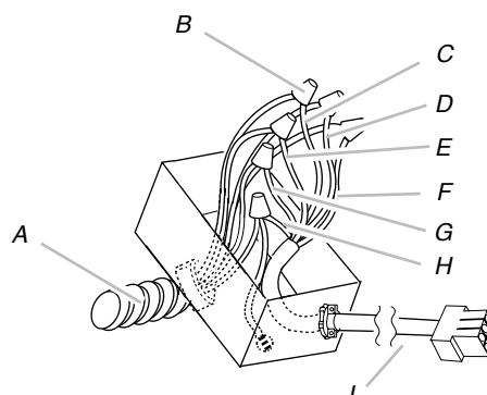
A. Décharge de traction B. Fil listé UL C. Fils noirs D. Fils blancs E. Fils rouges F. Fils bleus G. Fils gris H. Fils vert (ou jaune / vert) et vert / jaune I. Prise électrique du moteur câble
