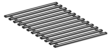
Bottom Slat 997 x 45 x 18mm
