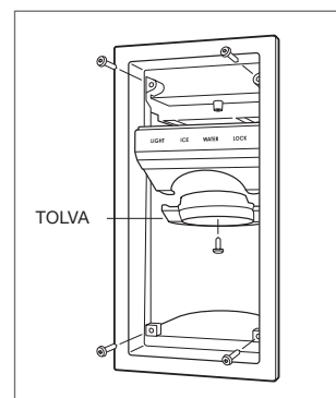
Retirada del bisel del dispensador
