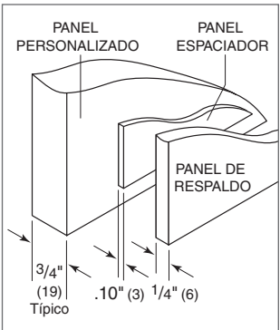
Vista posterior del montaje del panel
