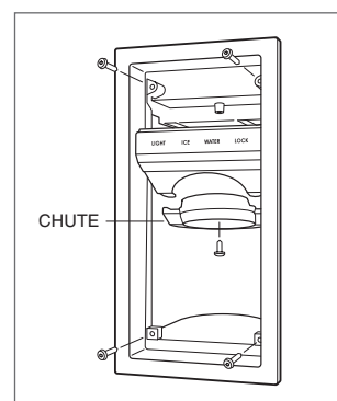
Enlèvement de la lunette du distributeur
