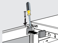
Pasador de la bisagra/ retenedor del pasador de la bisagra
