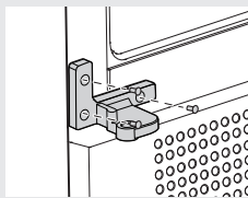
Bisagra inferior del lado izquierdo
