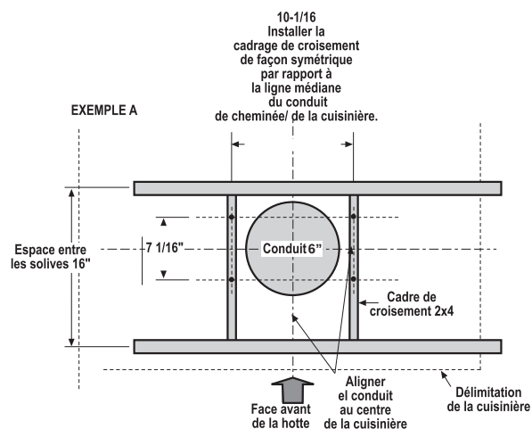
Vue du dessus – Solives du plafond parallèles à la face avant de la hotte
