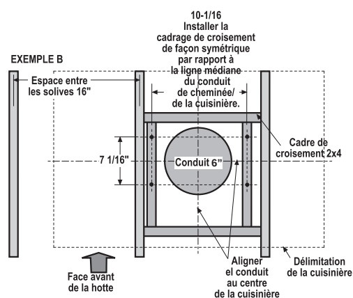
Vue du dessus – Solives du plafond perpendiculaires à la face avant de la hotte
