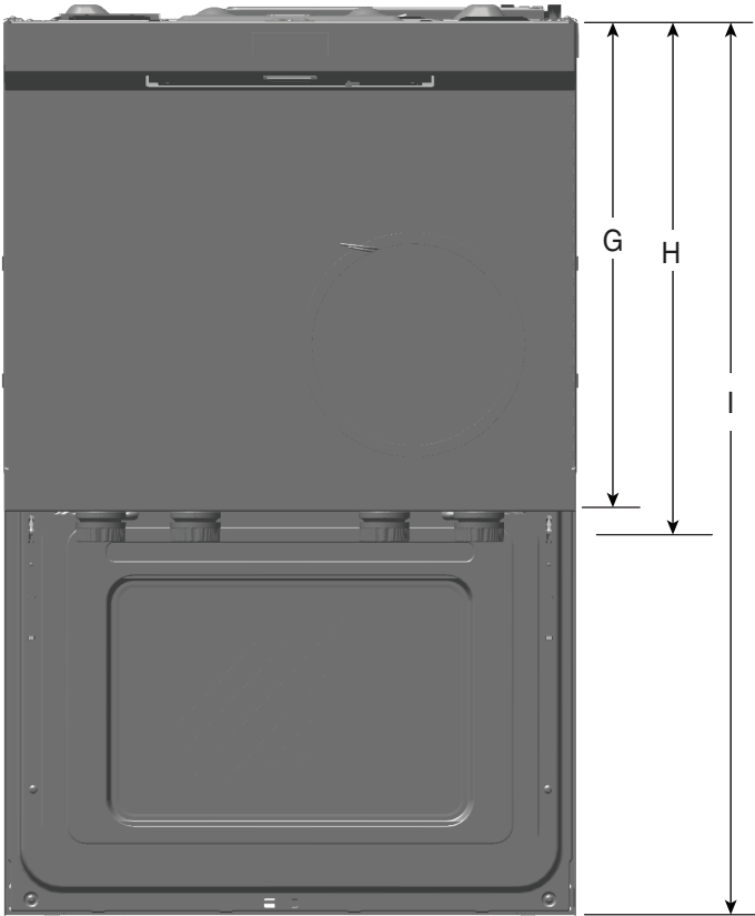
VISTA SUPERIOR
