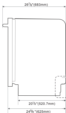
Vue latérale Série DW80N3030
