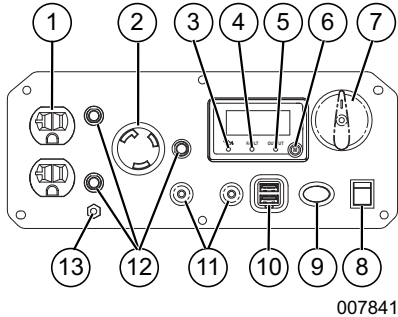
Figure 2-2. Panneau de commande
