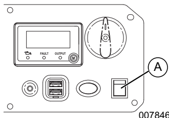
Figure 3-4. Commutateur « Arrêt/ON/START »
