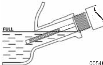
Imagen 2-11. Rango de funcionamiento seguro
