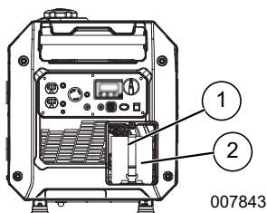
Imagen 2-8. Conexión de la batería
