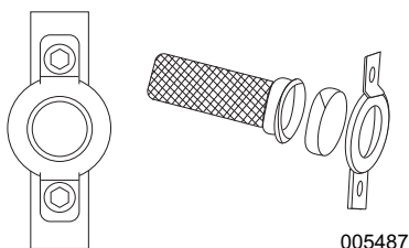
Imagen 4-8. Pantalla del supresor de chispas
