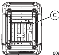
Imagen 4-4. Retirar la tapa de goma del drenaje de aceite
