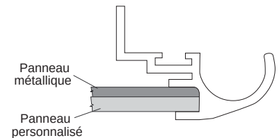
Panneau encastré
