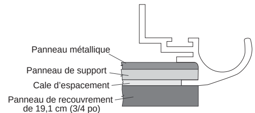
Panneau encastré
