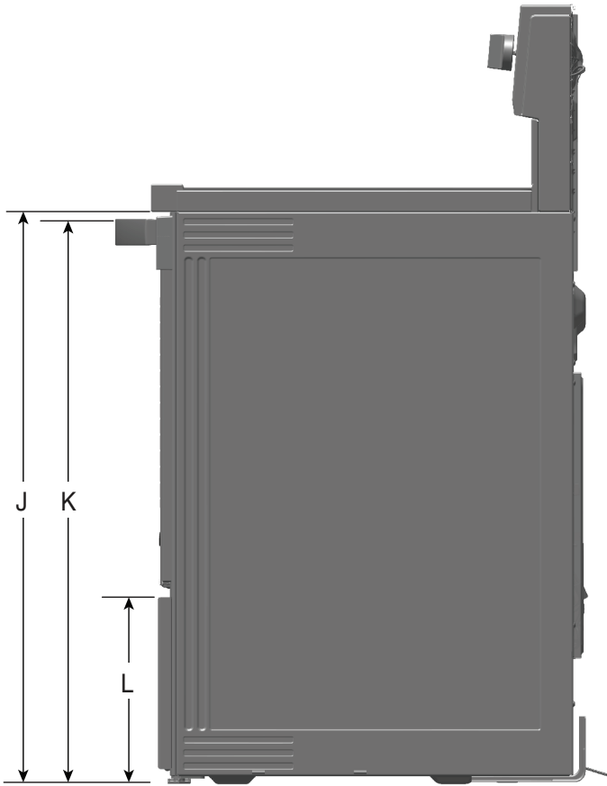
VISTA LATERAL
