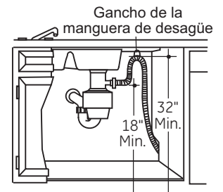
Instalación del eliminador de desechos
