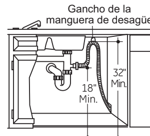
Instalación de la T de desechos Figura AC
