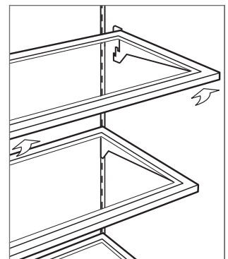
Retrait d'une tablette en verre.
