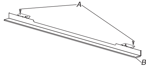
A. Tornillos Phillips (2), solo 2 tornillos para el tamaño de 27" (68,6 cm) B. Deflector (1)
