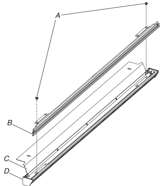
A. Tornillos n.º 8-18 x 1/4" (6,4 mm) B. Deflector C. Pieza superior del ducto de ventilación D. Pieza inferior del ducto de ventilación
