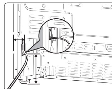
Ubicación del cable de alimentación
