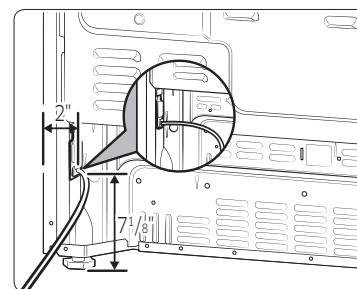
Emplacement du cordon d'alimentation
