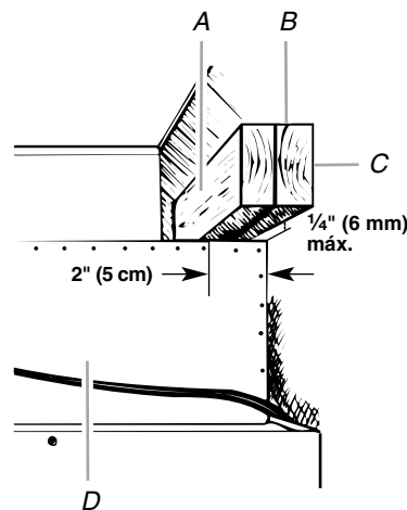
A. Tablero central \frac{1}{4} " (6,35 mm) como máximo arriba del refrigerador
