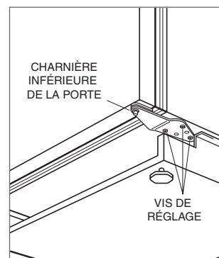
Charnière inférieure de la porte.
