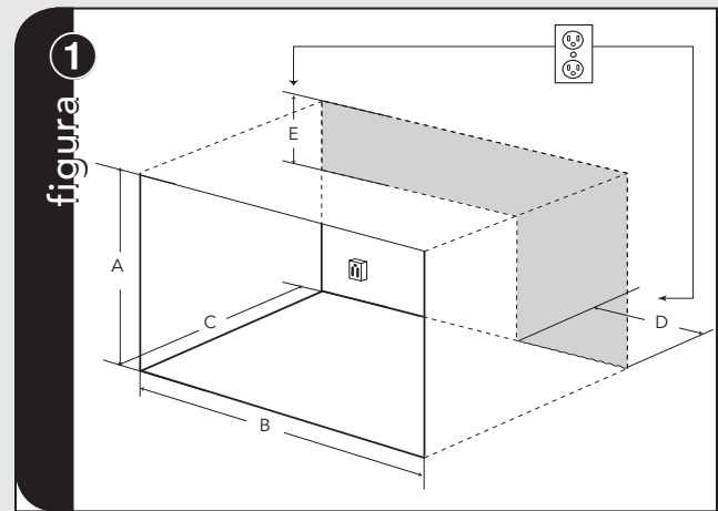
Dimensiones de los recortes para montaje en superficie
