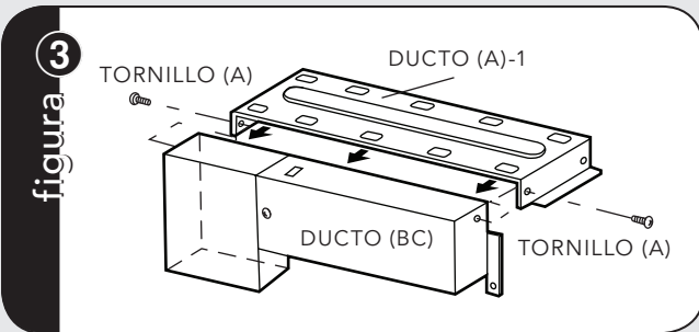
ENSAMBLAJE DEL DUCTO DE ESCAPE: Coloque el DUCTO (A)-1 en la parte superior del horno insertando el extremo del conjunto del DUCTO (BC) en el borde de retención del DUCTO (A)-1. Ajuste dos TORNILLOS (A), asegurando el DUCTO (A)-1 al conjunto del DUCTO (BC). Vea la figura 3.
