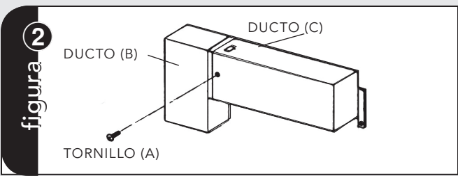
ENSAMBLAJE DEL DUCTO DE ESCAPE: Inserte el extremo del DUCTO (B) en el borde de retención del DUCTO (C). Asegúrelos usando un TORNILLO (A) incluido en el juego. Vea la figura 2.
