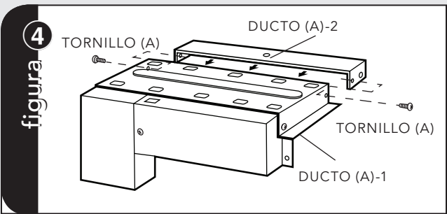
ENSAMBLAJE DEL DUCTO DE ESCAPE: Coloque el DUCTO (A)-2 en la parte superior del horno e insértela en el sostener labios de DUCTO (A)-1. Asegure el DUCTO (A)-2 a DUCTO (A)-1 utilizando dos TORNILLOS (A) incluidos. Vea la figura 4.
