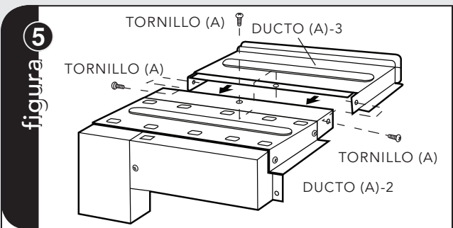
ENSAMBLAJE DEL DUCTO DE ESCAPE: Coloque el DUCTO (A)-3 en la parte superior del horno e insértela en el DUCTO (A)-2. Asegure el DUCTO (A)-3 utilizando tres tornillos (A) incluidos. Vea la figura 5.
