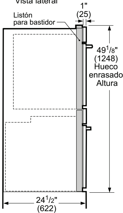
Vista lateral
