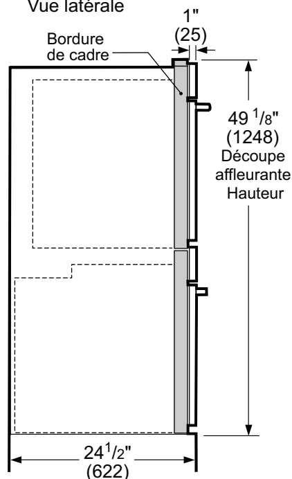
Vue latérale
