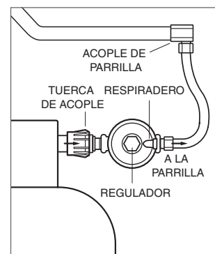
Conexión del cilindro de gas propano líquido
