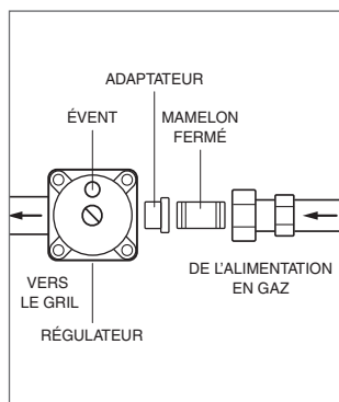
Régulateur du gaz naturel
