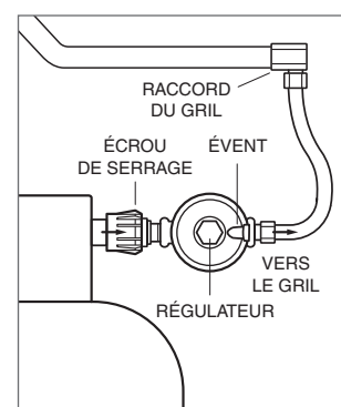
Connexion de la bonbonne de GPL
