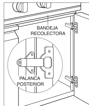
Retire la puerta del carro
