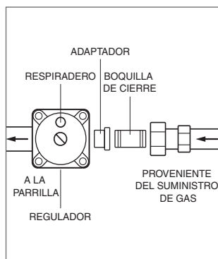
Regulador de gas natural
