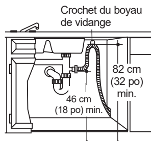
Installation avec raccord en T Figure AC
