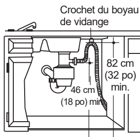
Installation avec broyeur à déchets
