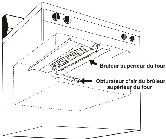
Fig. 19 - Emplacement des brûleurs du four
