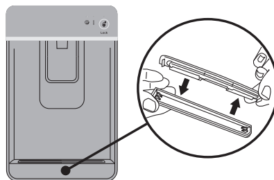
Nettoyage du plateau d'égouttage
